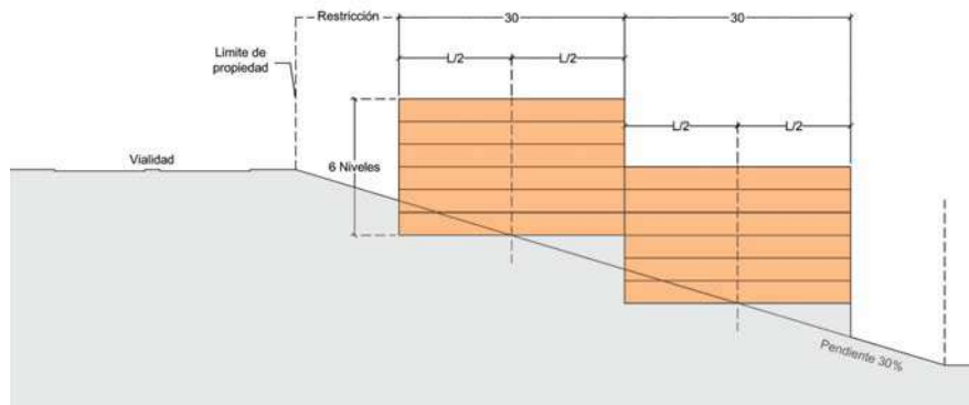
Ilustración 267: Desplante de módulos de longitud mayor a 30m con pendiente descendente.
