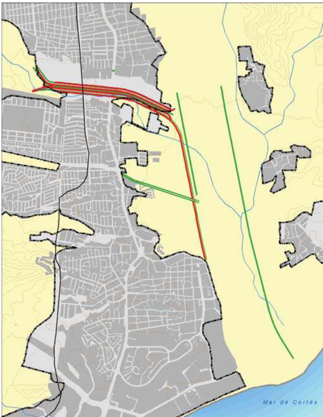
Ilustración 100: Canalización de arroyos en San José del Cabo. Fuente: Dirección General de Asentamientos Humanos y Obras Públicas
