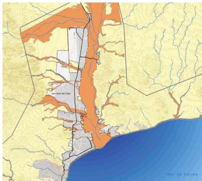
Ilustración 31: Esquema de flujos de lodos San José del Cabo En base a datos de Atlas de Riesgo 2007
